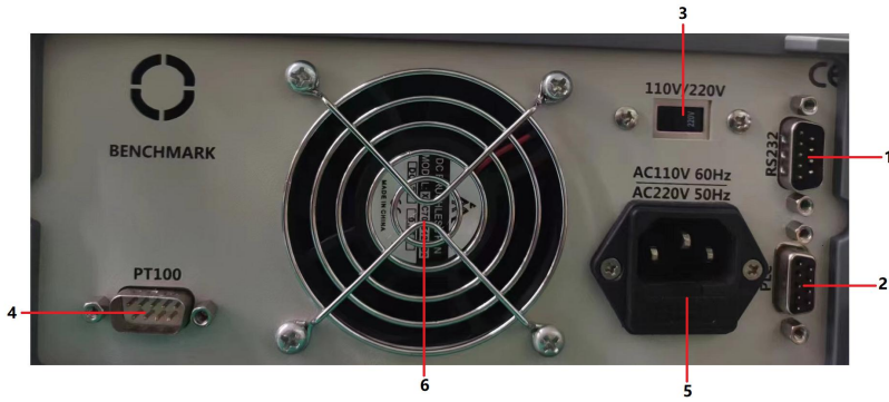
图 2-2 后面板说明
